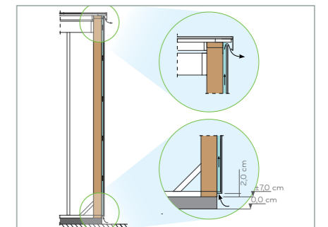
Ingebouwd ventilatiesysteem
